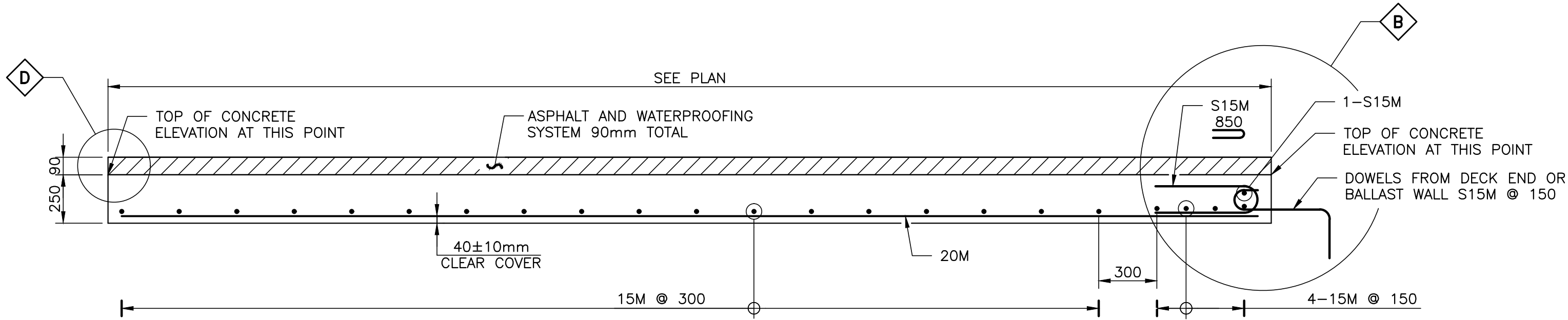
LONGITUDINAL SECTION SCALE 1:20
