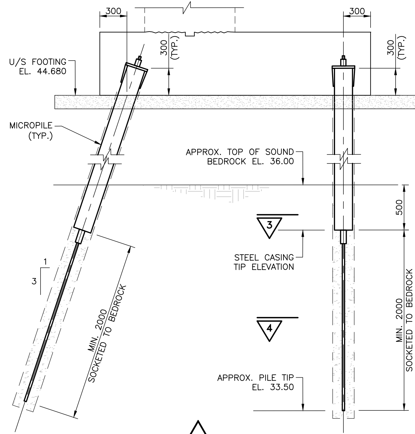
SECTION 1:25
