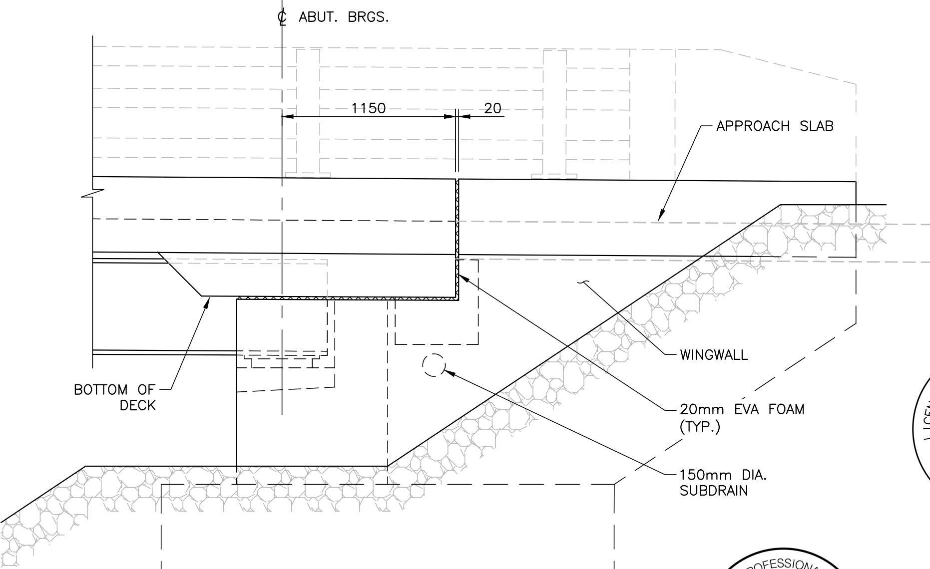
1 SECTION 1:25
