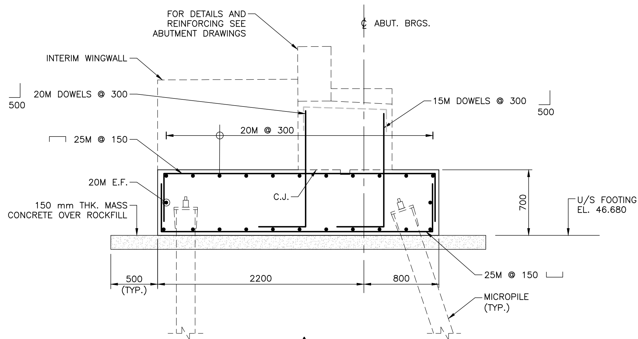
SECTION 1:25
