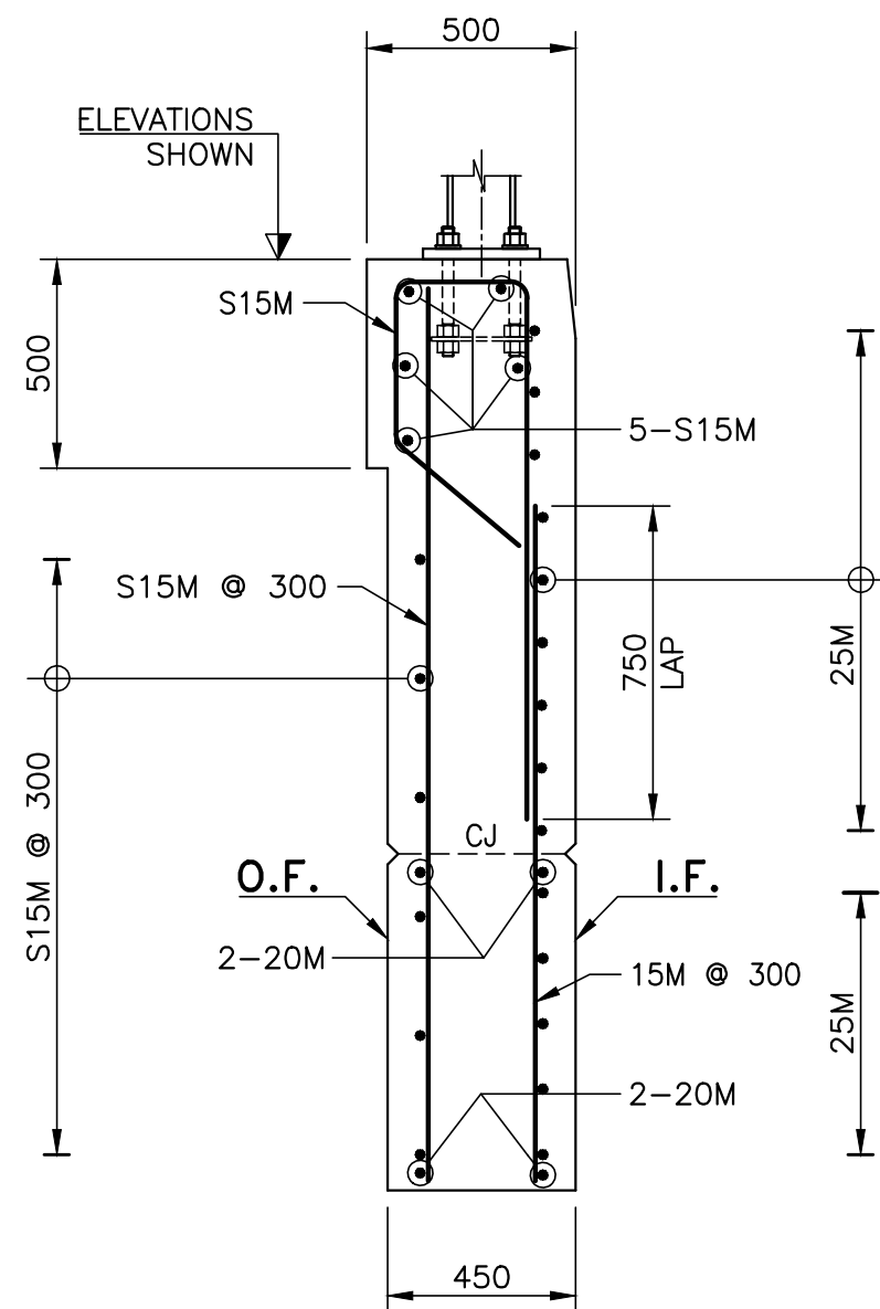
2 SECTION 1:20
