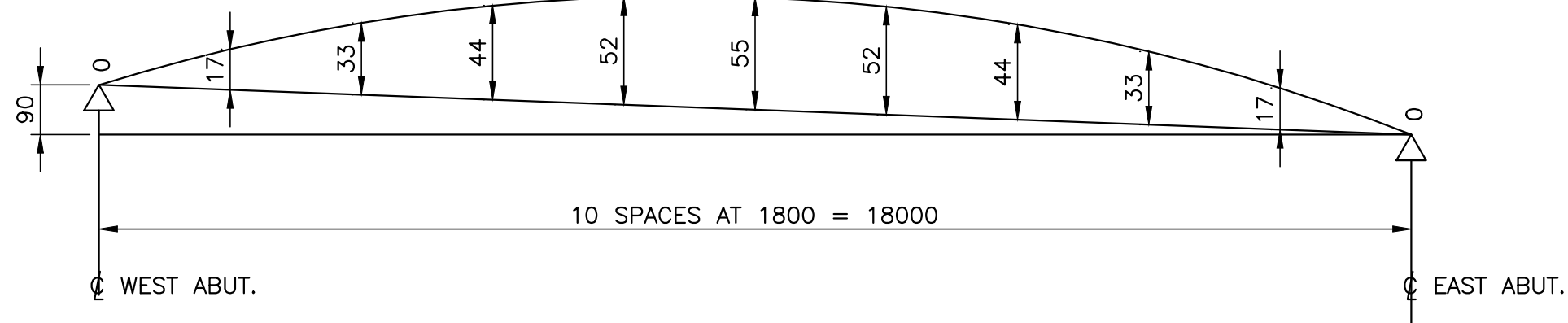
RELAXED CAMBER DIAGRAM N.T.S.
