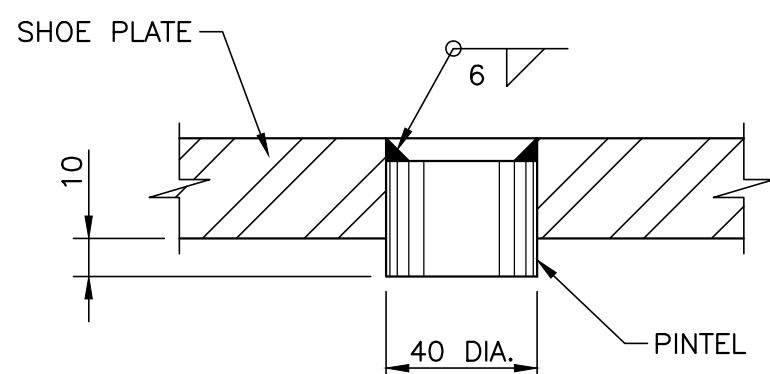
PINTEL DETAIL 1:2
