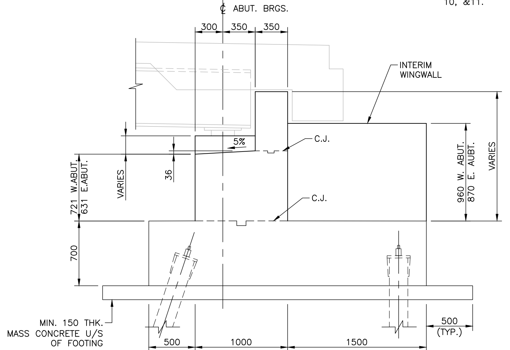
1 SECTION 1:25
